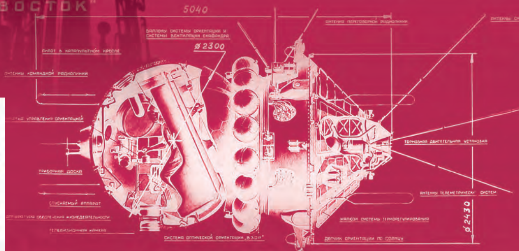
Внутреннее устройство космического корабля «Восток». Из личного фонда А.В. Палло. РГАНТД. Ф. 107. Оп. 2-10. Д. 176. Л. 1
